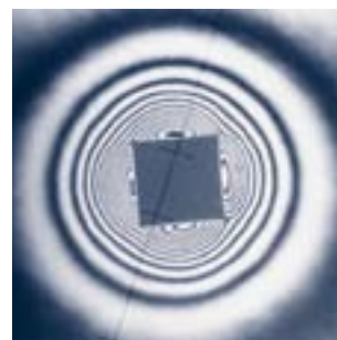
Lichtinterferenzbild eines Vickerseindrucks Interference picture of a Vickers indentation
